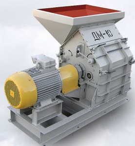
Дробилка молотковая ДМ-10
